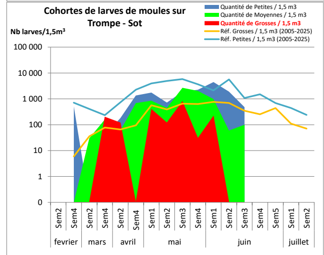
Quantités de larves aux stades « Petites », « Moyennes » et « Grosses », observées en 2026 et moyennes de référence (« Petites » et « Grosses ») observées pour la même période sur le site de Boyard (2005-2025) et le site de Trompe-Sot (2011 à 2025), pour 1,5 m 3 .
