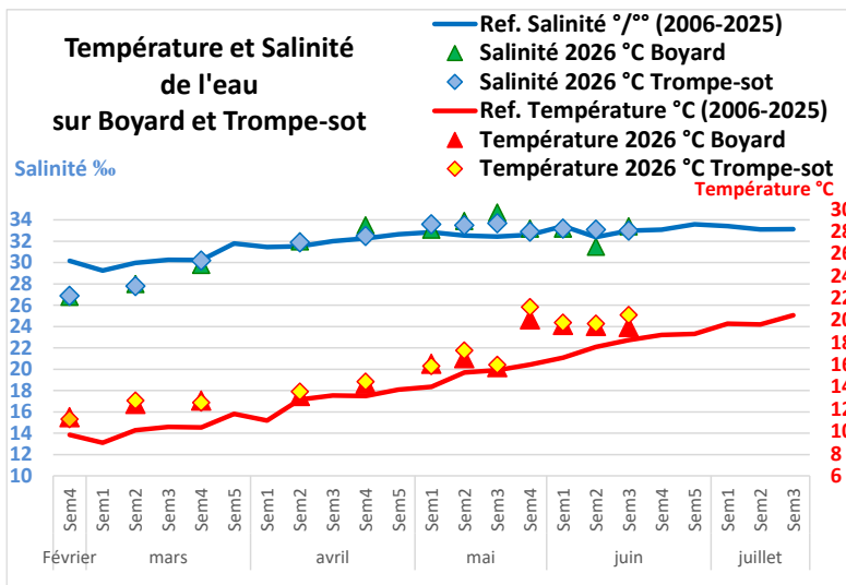
Évolution de la température de l'eau (°C) et de la salinité (g/l, ou ‰) sur le site de Boyard et Trompe-Sot, comparées aux références : moyennes de 2005 à 2025.
