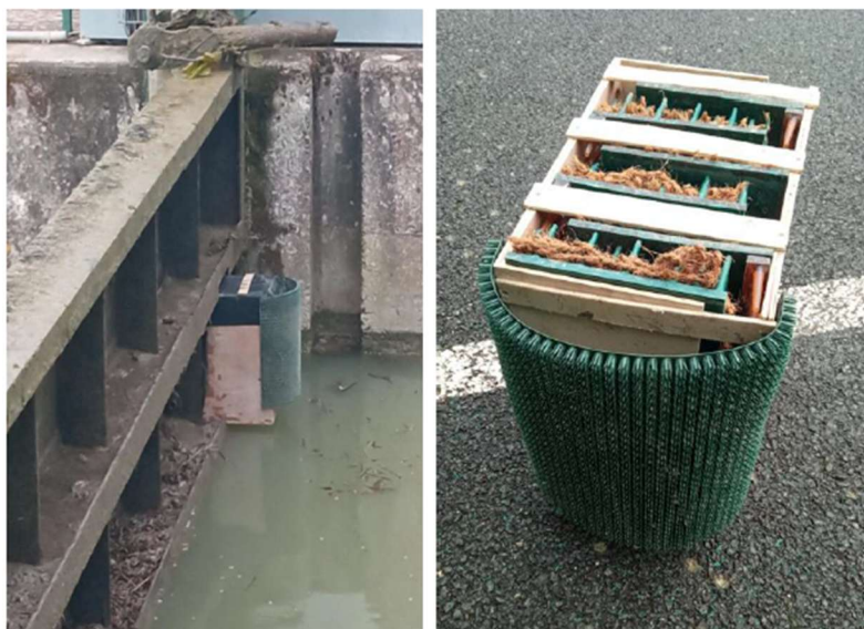
Figure 61 : Présentation de l'équipement complémentaire (« boîte » en version avec plots et support en fibres de coco) et de son implantation sur la lumière
