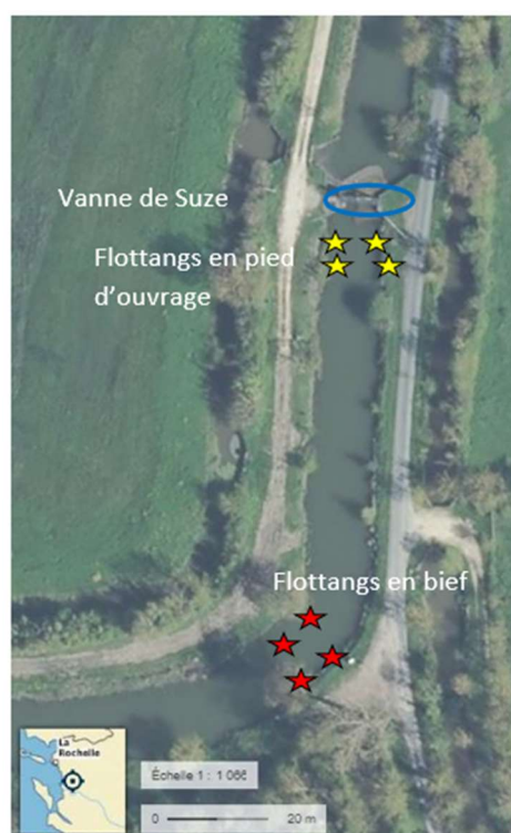
Figure 63 : Site de Suze et disposition des flottangs
